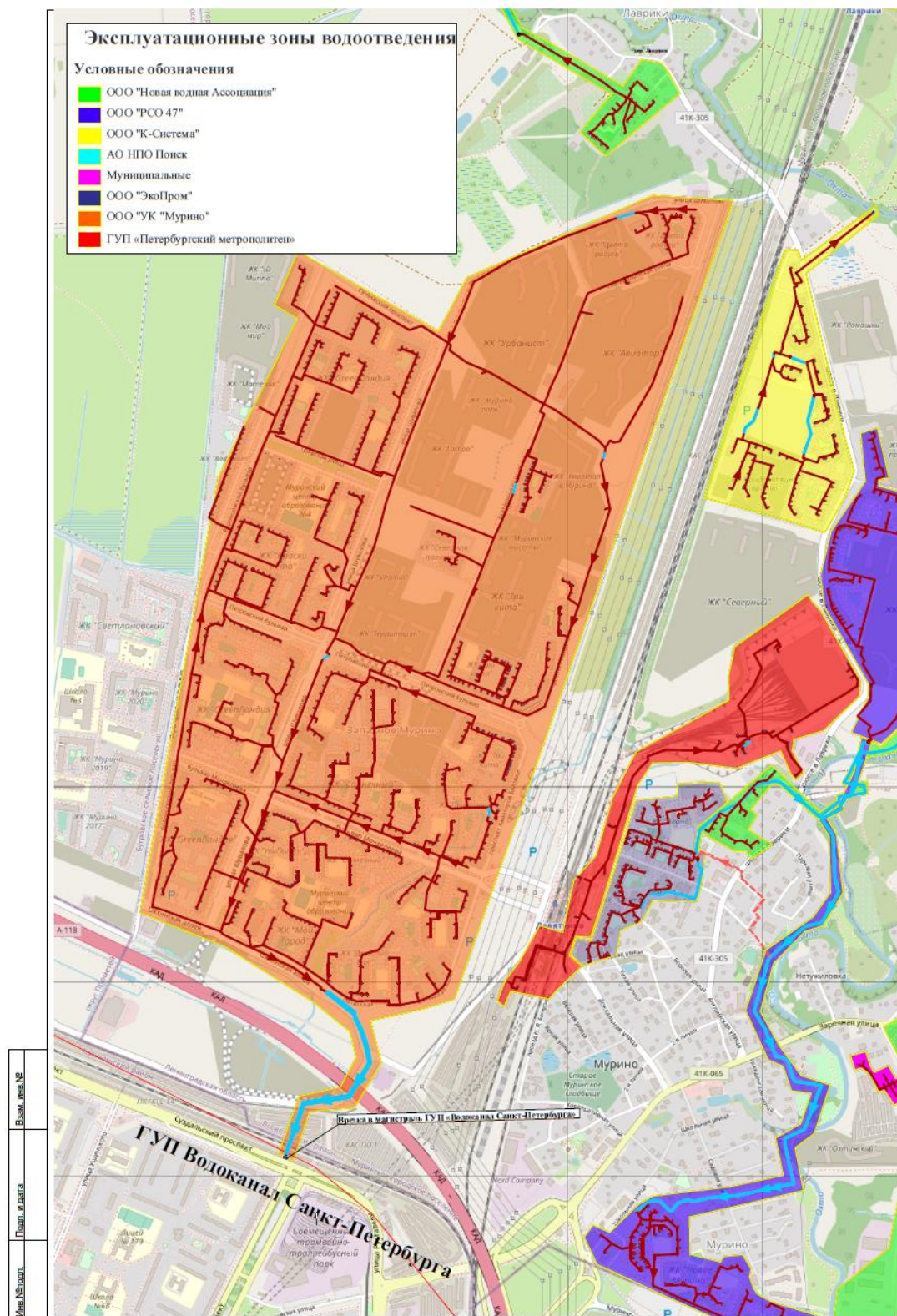
Рисунок 42 — Эксплуатационная зона водоотведения ООО «УК «Мурино»
