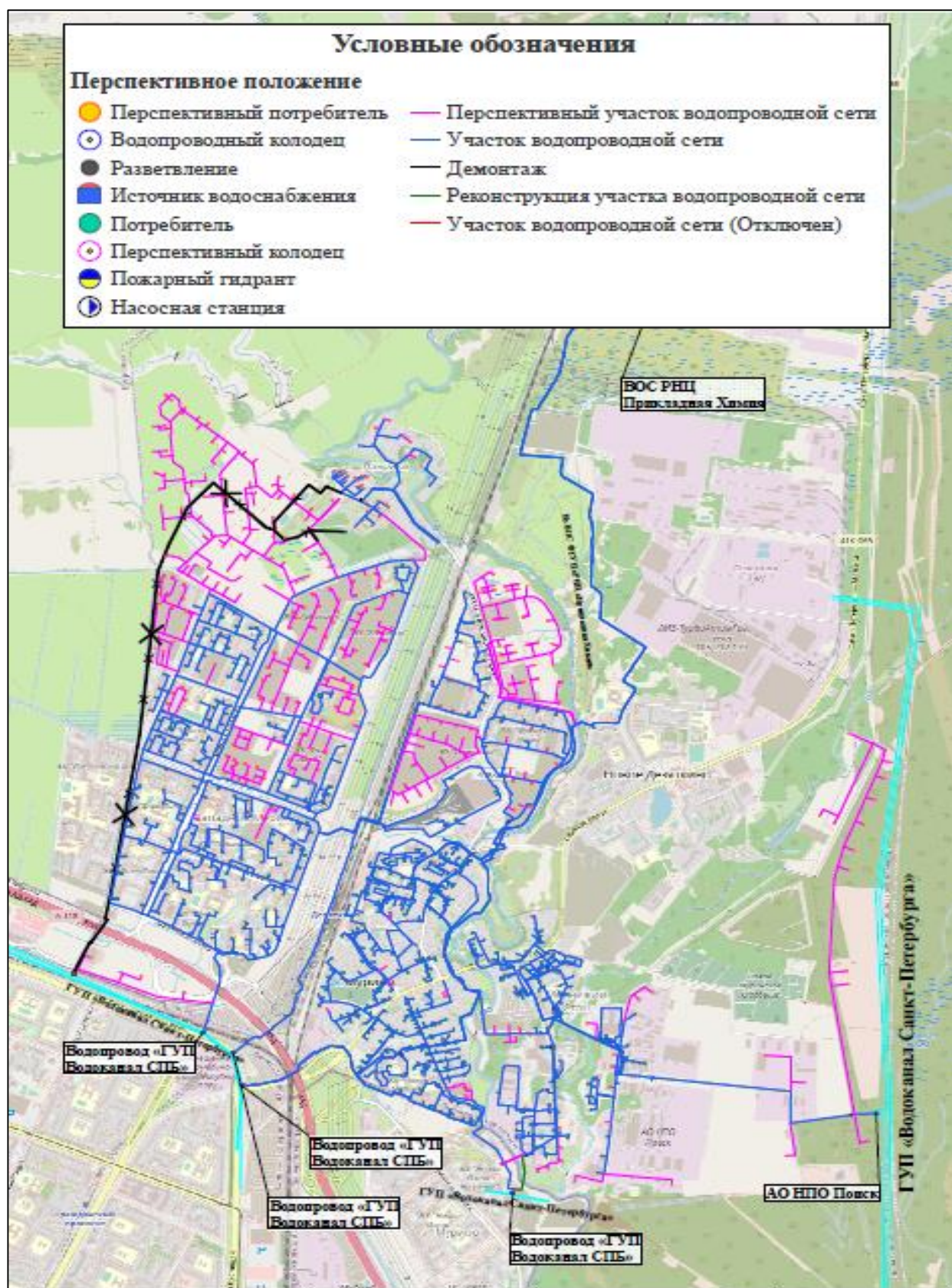
Рисунок 39 —Перспективная схема водоснабжения Муринского городского поселения
