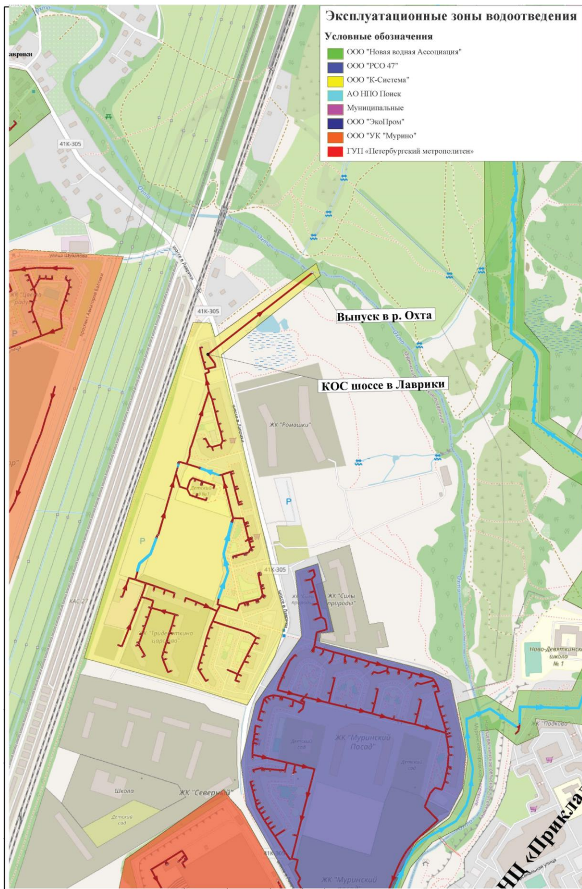
Рисунок 48 — Эксплуатационная зона водоотведения ООО «К-Система»
