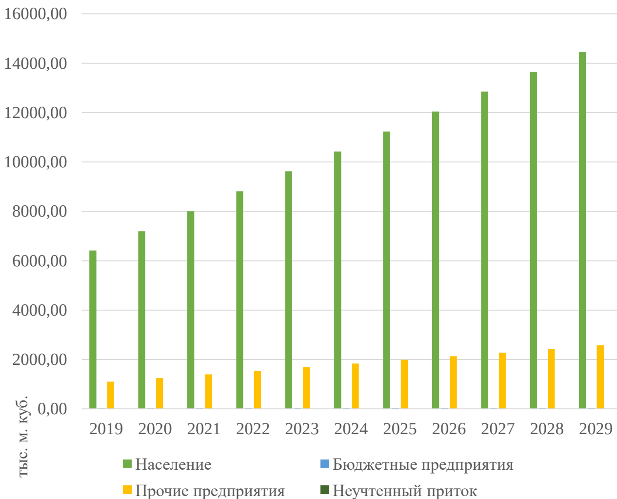
Рисунок 73 — Прием сточных вод от абонентов за 2019-2029 годы (при проектировании СВО)
