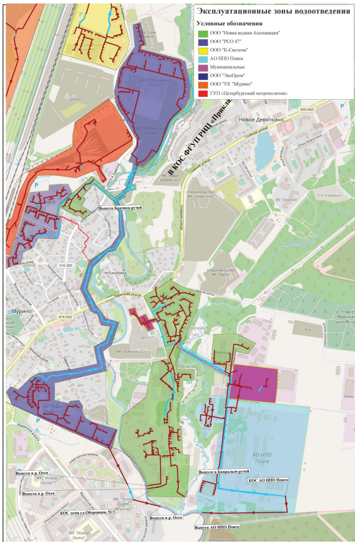
Рисунок 43 — Эксплуатационная зона водоотведения ООО «РСО 47»
