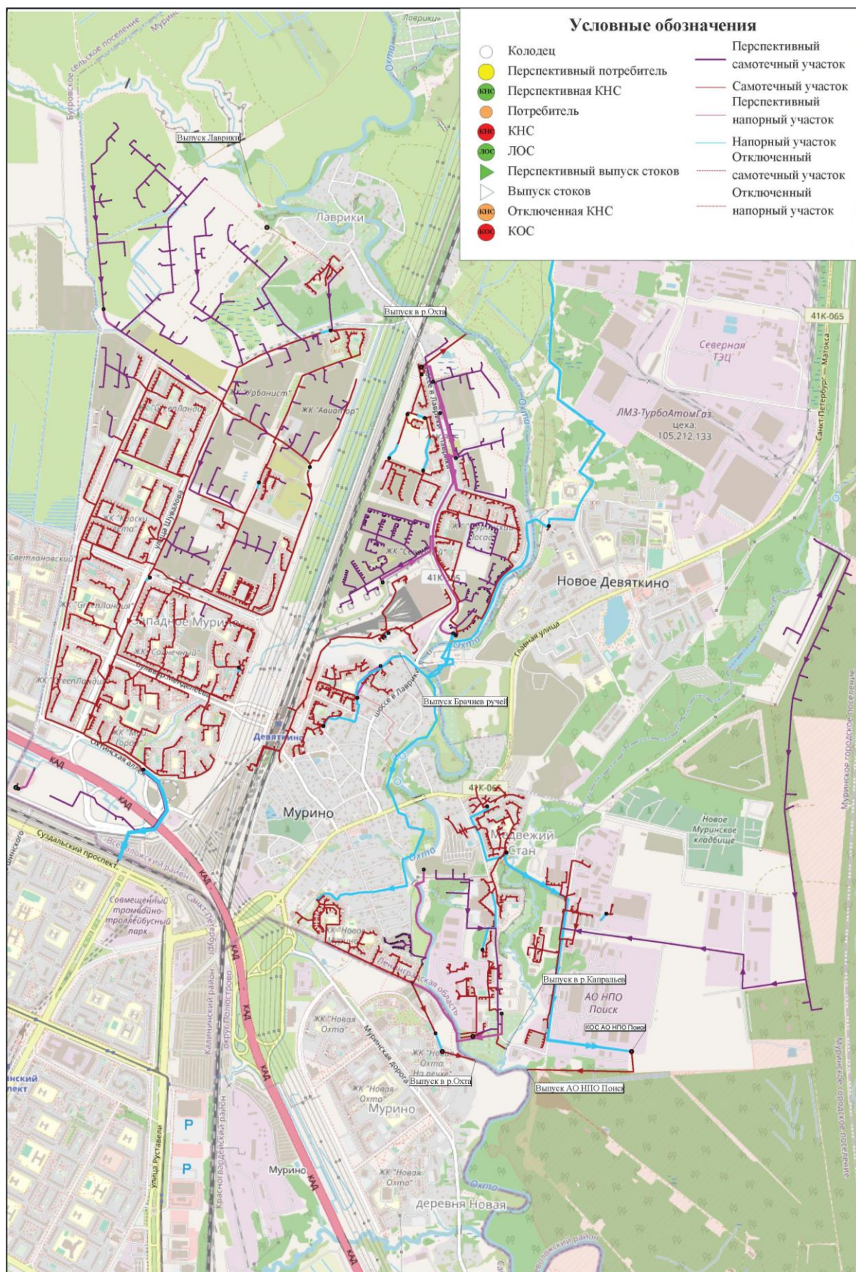
Рисунок 72 — Перспективная схема водоотведения Муринского городского поселения
