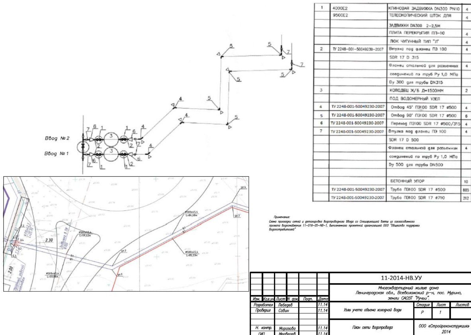
Рисунок 38 — Схема расположения и мест отбора проб холодной воды
