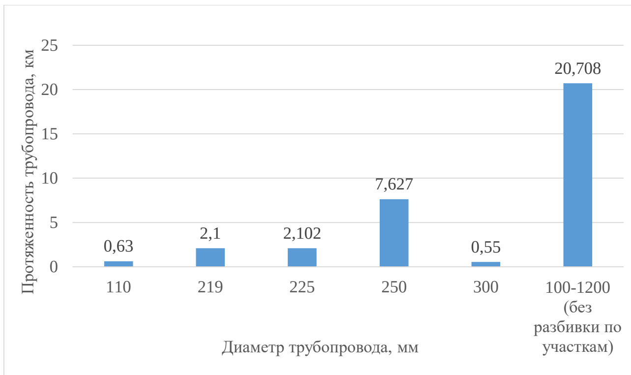
Рисунок 54 — Долевое распределение водопроводных сетей Муринского ГП по диаметрам трубопроводов
