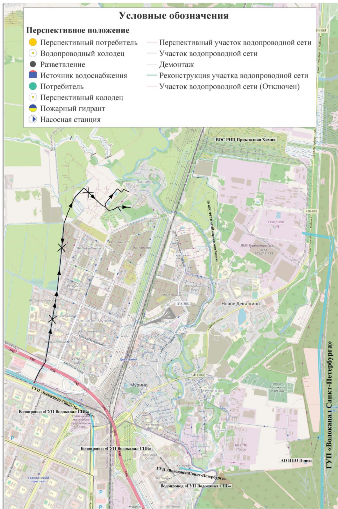
Рисунок 39 —Перспективная схема водоснабжения Муринского городского поселения
