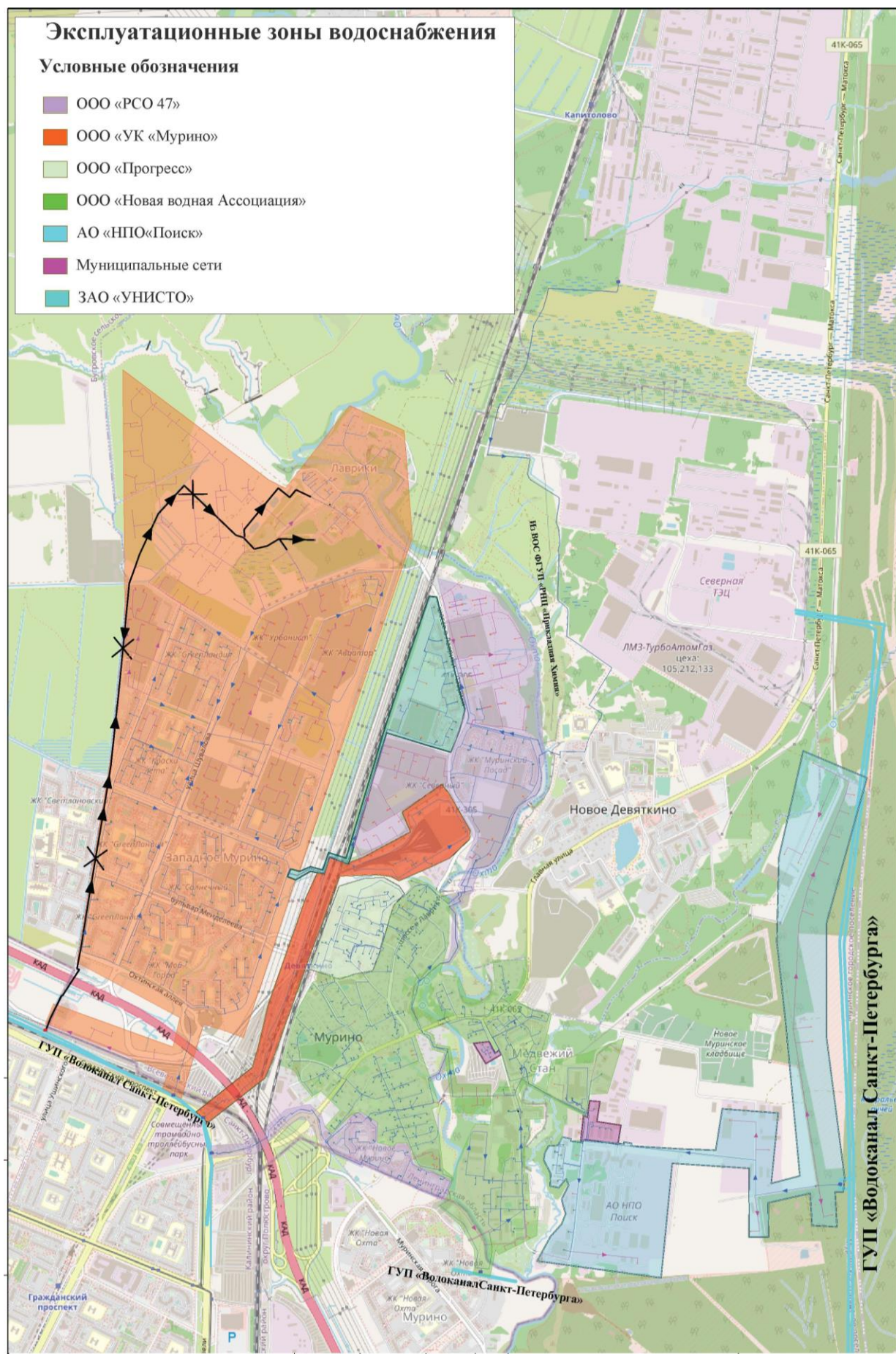
Рисунок 2 — Эксплуатационные зоны водоснабжения
