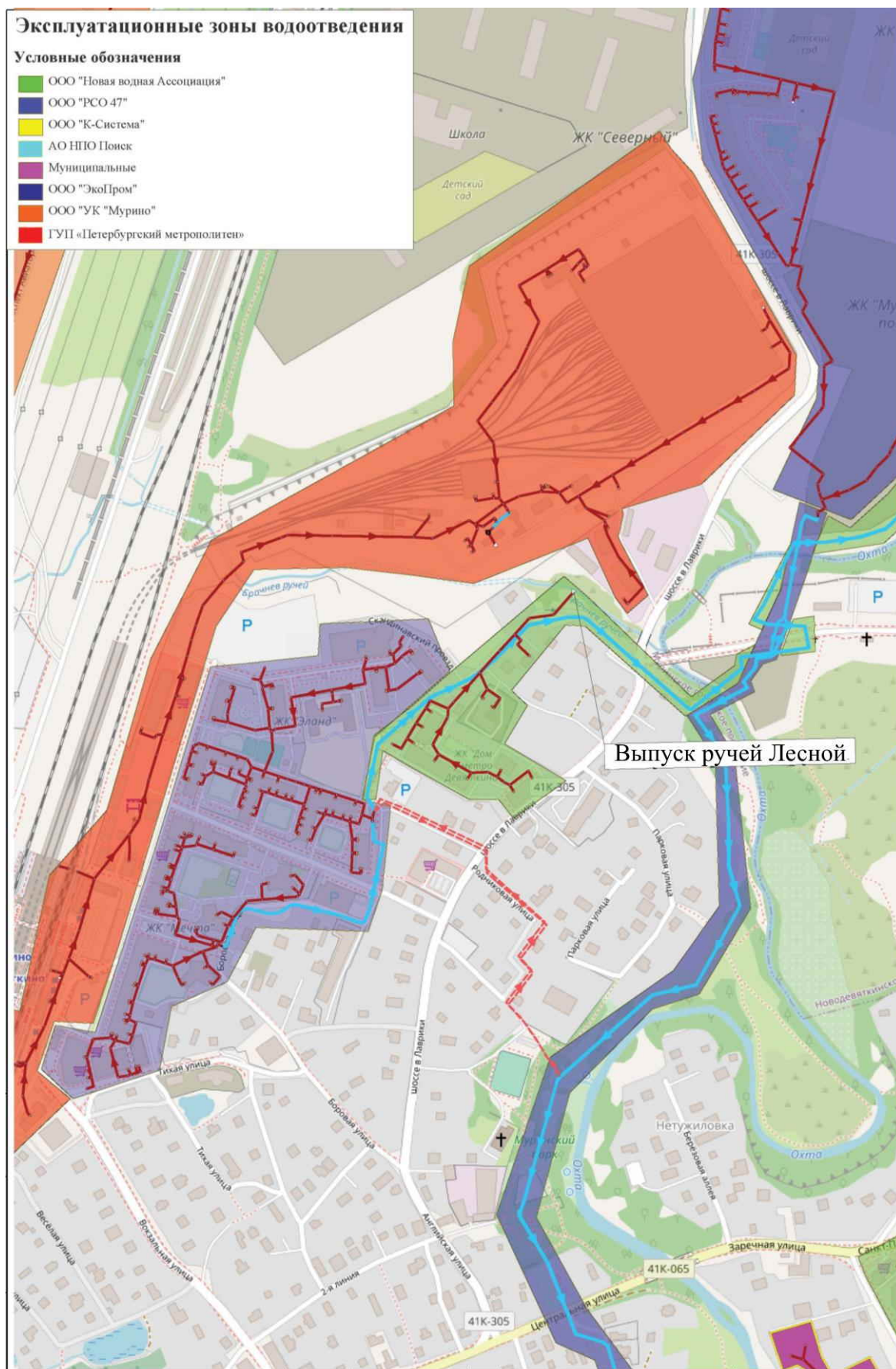
Рисунок 49 — Эксплуатационная зона водоотведения ООО «Новая Водная Ассоциация»
