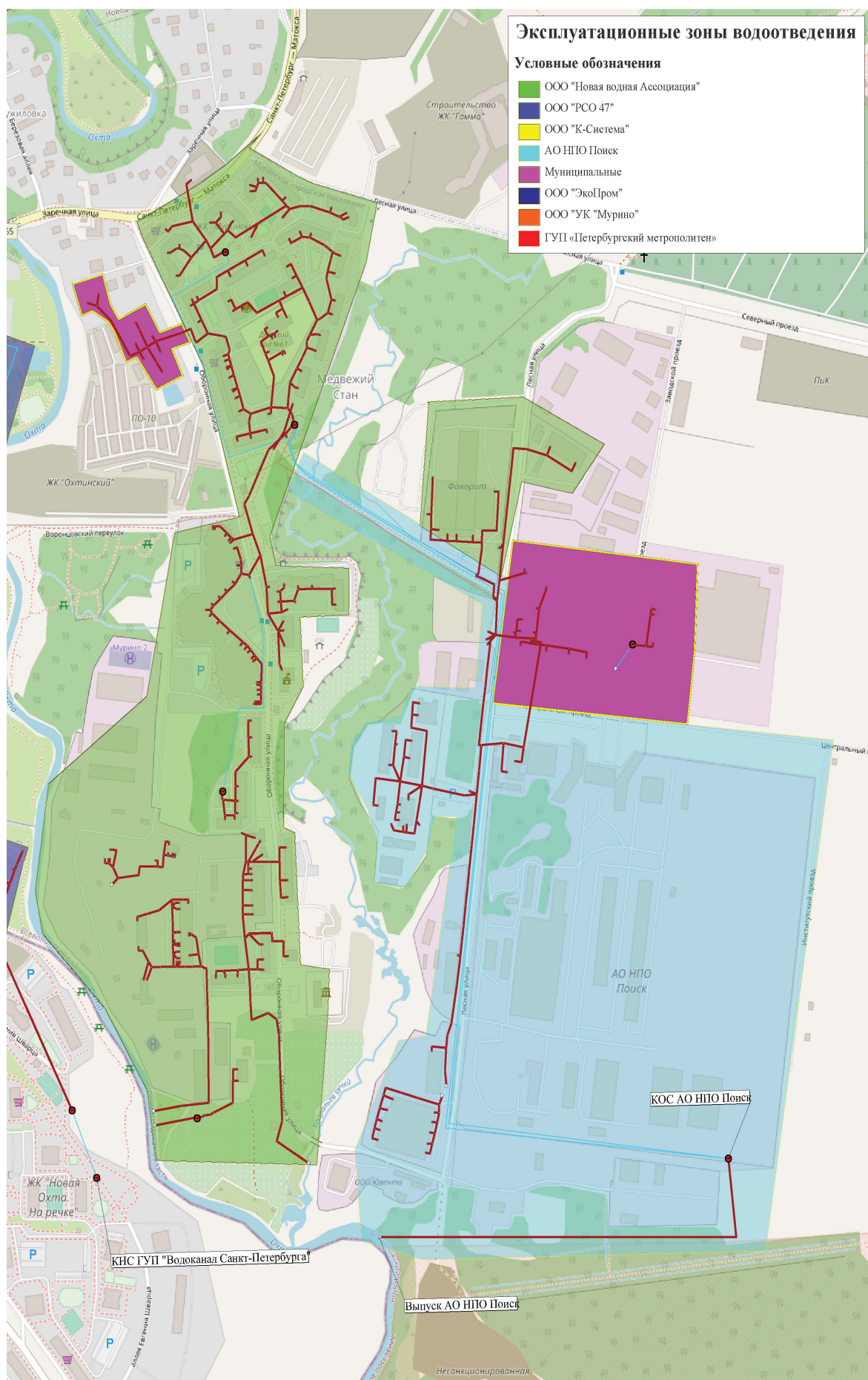
Рисунок 50 — Муниципальные канализационные сети
