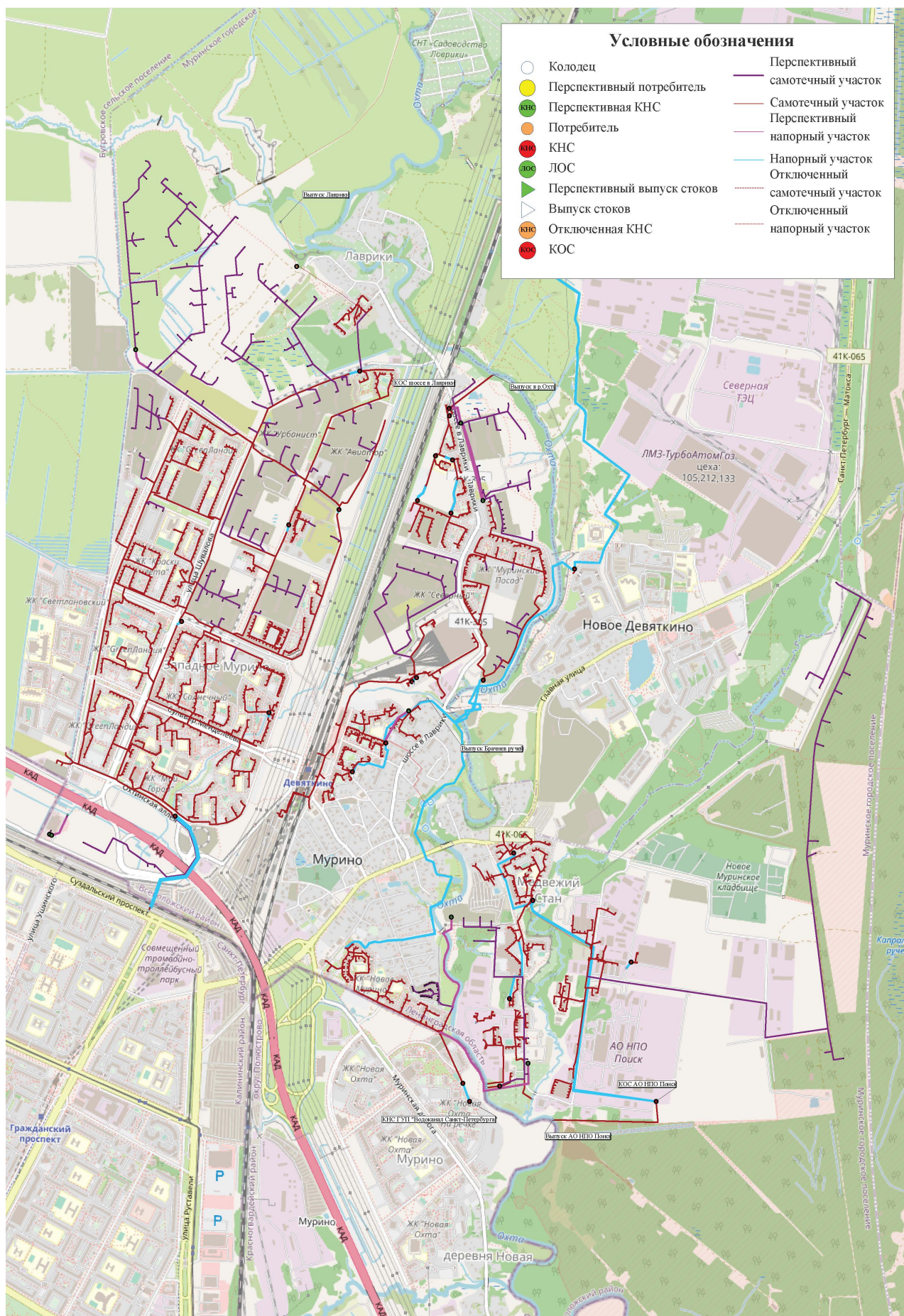
Рисунок 72 — Перспективная схема водоотведения Муринского городского поселения
