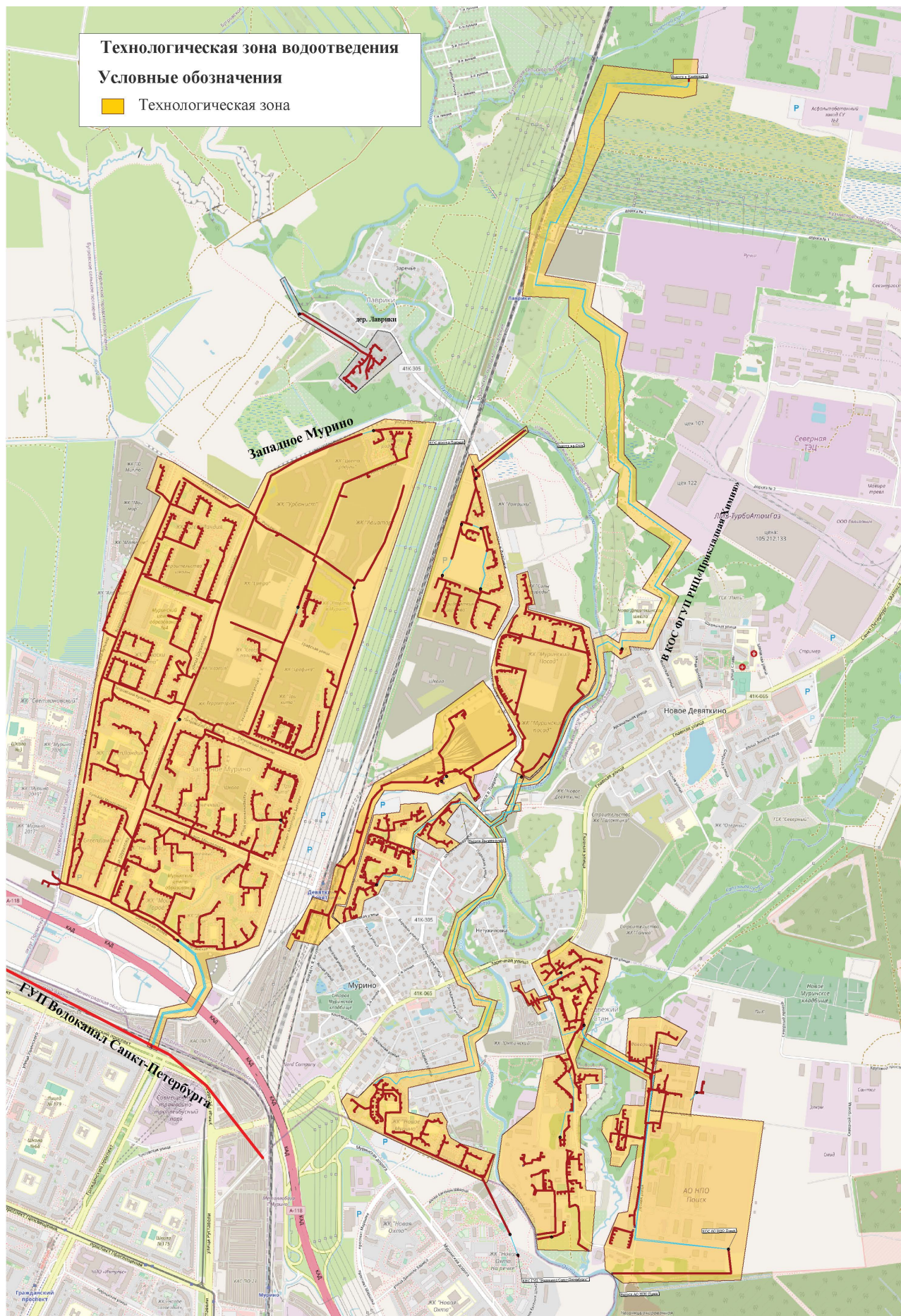
Рисунок 51 — Технологическая зона водоотведения г. Мурино
