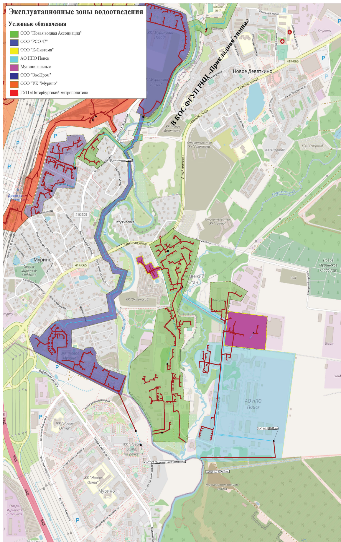
Рисунок 44 — Эксплуатационная зона водоотведения ООО «Новая Водная Ассоциация», г. Мурино
